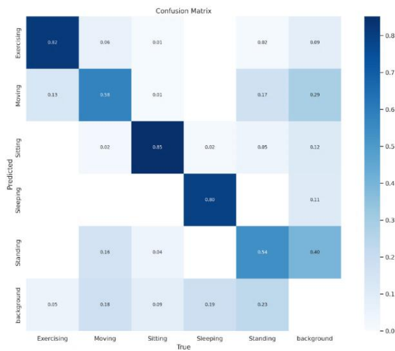
Fig. 14. YOLOv8x confusion matrix.
