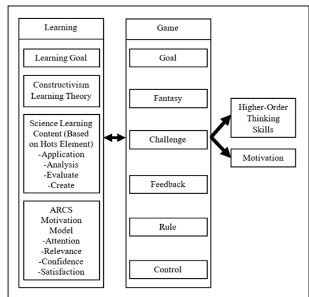
Fig. 5. PKBATDPS model.
