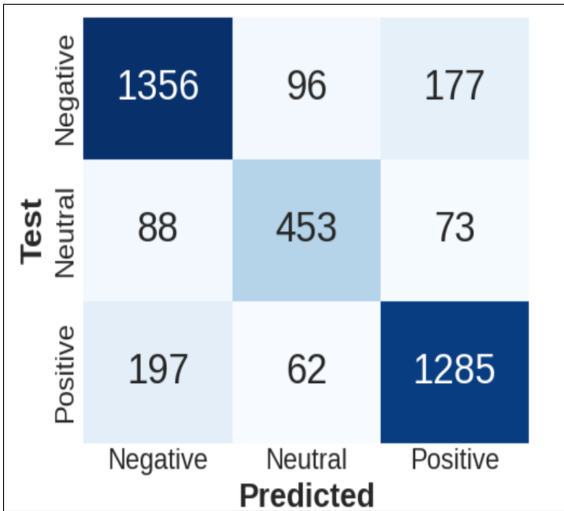
Fig. 11. CNN confusion matrix.
