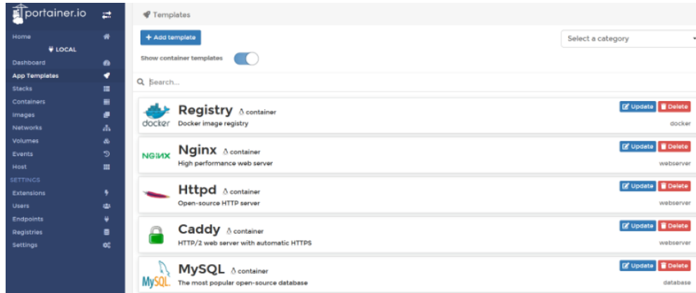
Fig. 6. App template.
