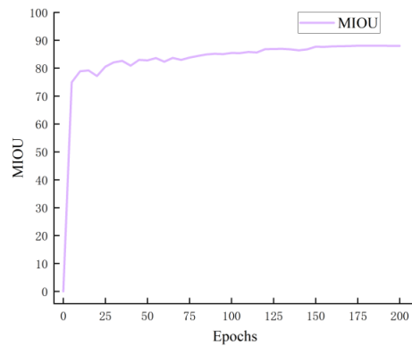
(b) MIOU.
