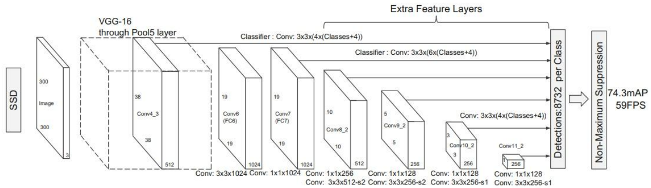
Fig. 1. SSD Model [28].
