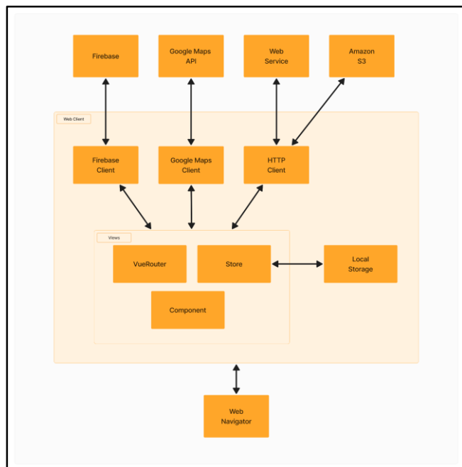
Fig. 4. Web architecture.
