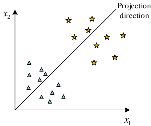
Fig. 1. LDA.
